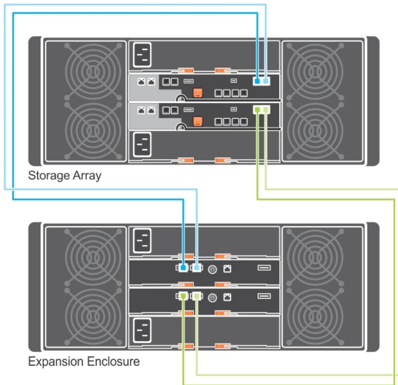
Abbildung 5. Einzelerweiterung-Diagramm
