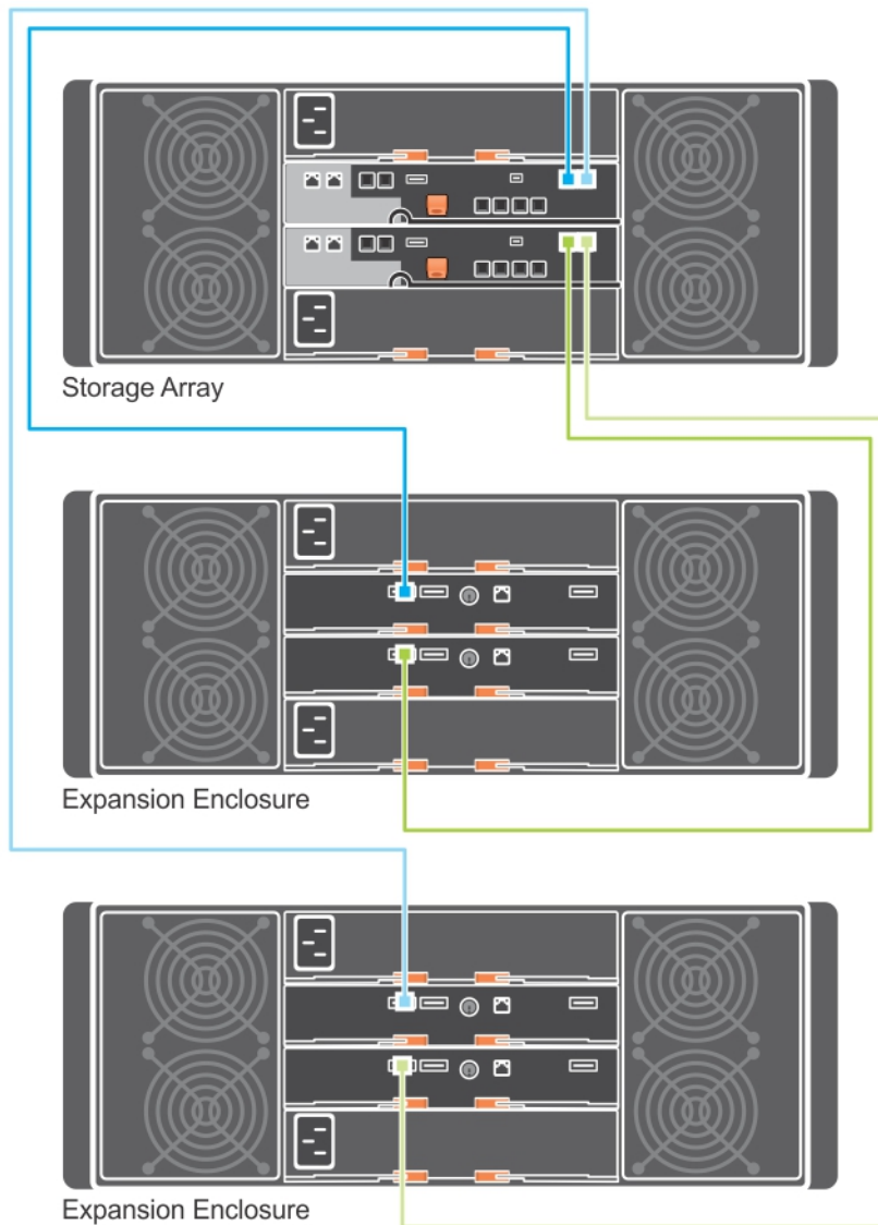
Abbildung 6. Dual-Erweiterung-Diagramm
